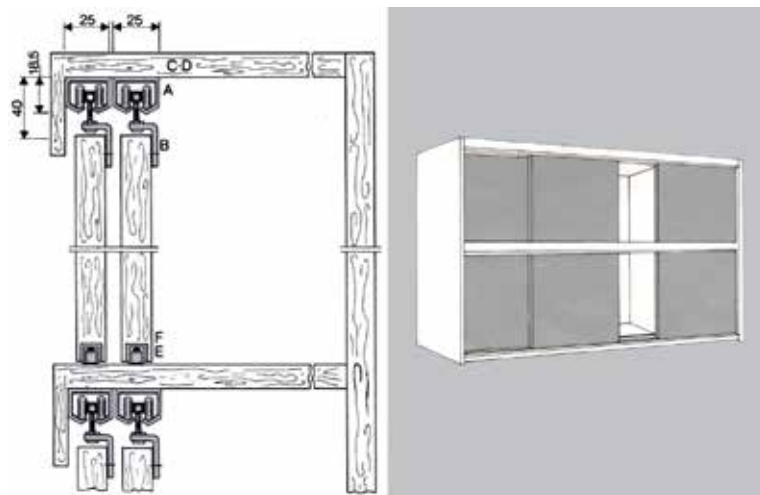
Schuifdeurbeslag type Omge 2032
