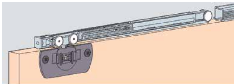
Demper voor Hawa schuifdeurbeslag type Clipo 16 Mixslide
