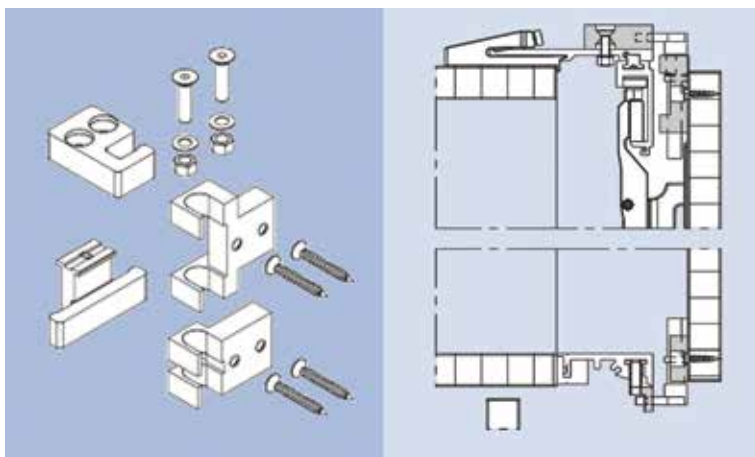
Aanslagset voor stangslot voor Hawa Folding Concepta 25
