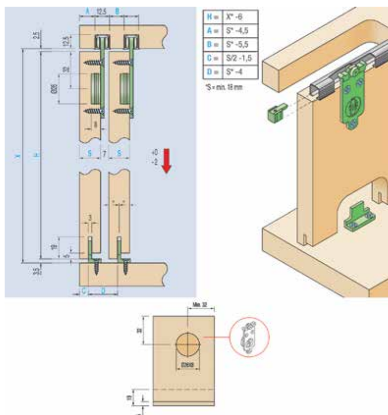
Schuifdeurbeslag type Sisco 900 Economic
